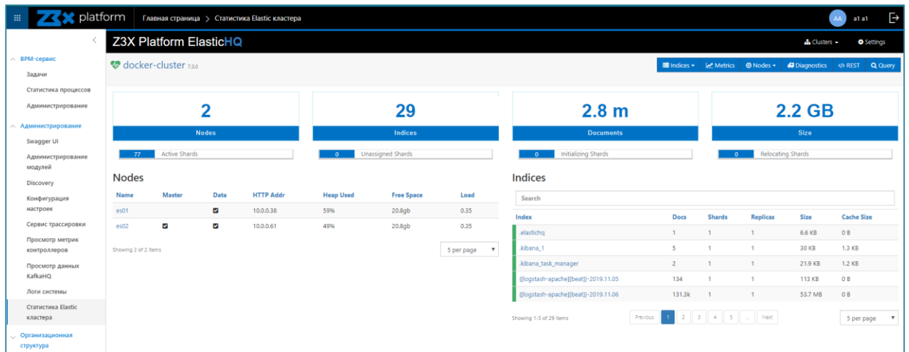
Рисунок 19 – Страница «Статистика Elastic кластера»
