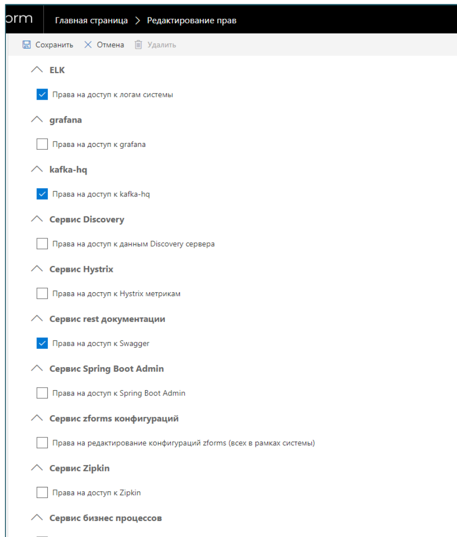
Рисунок 26 – Настройка прав системной роли
